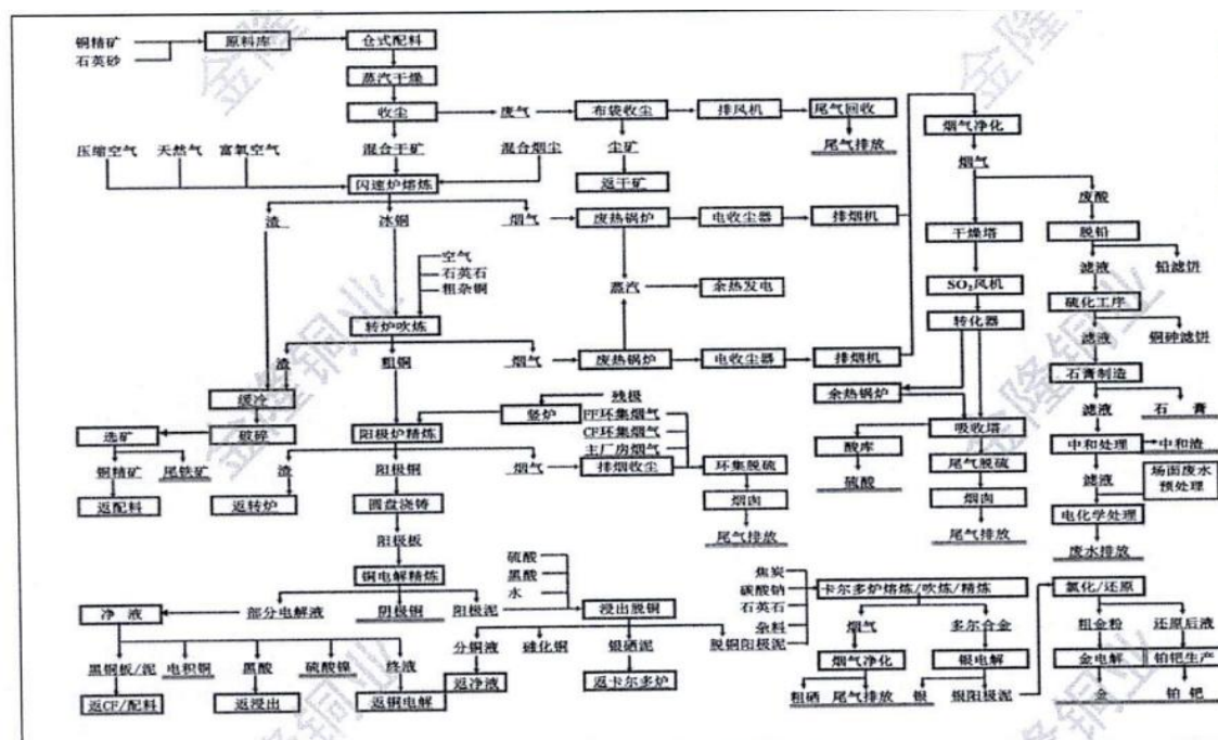
图 3-1 铜冶炼工艺流程图
